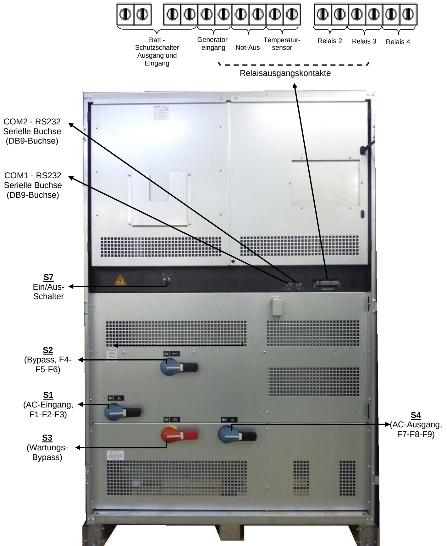
Abb. 1.3 a Schalter, Sicherungen und Schnittstellenanschlüsse 200 - 250 - 300 - 400 kVA
