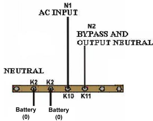
Ab. 2.2 Stromkabelanschluss 100-120-160 kVA
